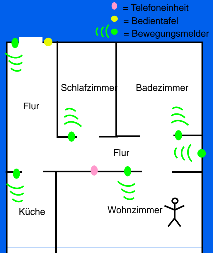
Schaubild: Aktivitätsmonitoring 13
